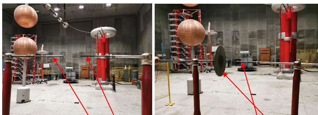
a) Sistem de electrozi vârf – vârf
